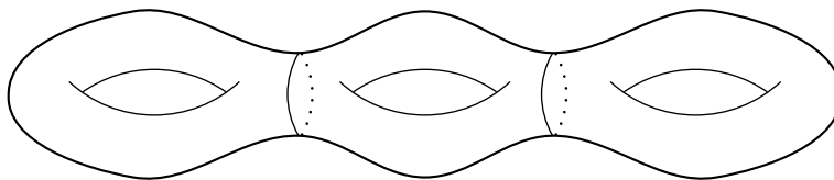
Slika I.2: Orientabilna ploskev roda g = 3
