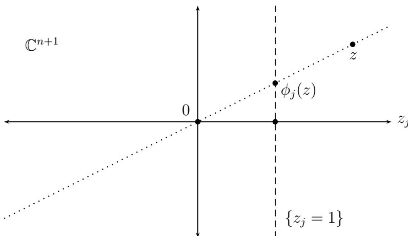
Slika I.1: Afine koordinate na \mathbb{CP}^n
