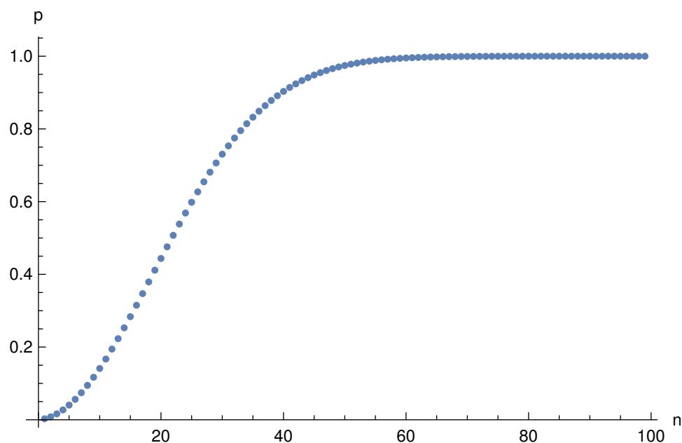
Slika 2: Verjetnost, da imata med n ljudmi vsaj dve osebi isti rojstni dan.
