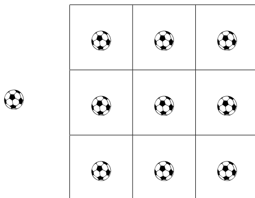
Slika 1: Deset žogic in devet škatel.
