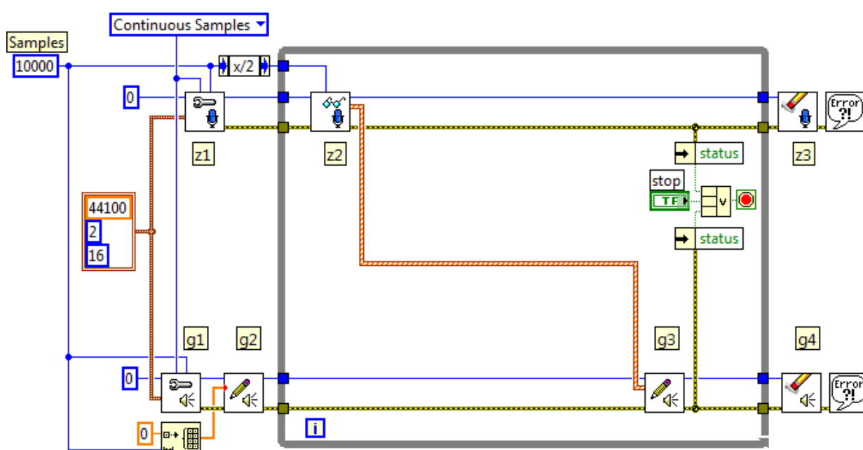
Slika 9: Zgled programa za neprekinjeno sočasno zajemanje in generiranje signalov z zvočno kartico
