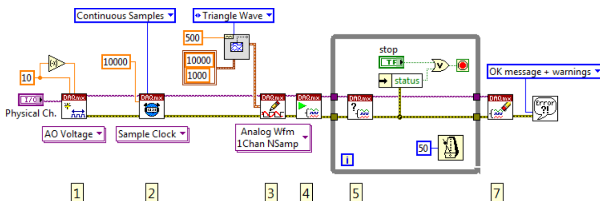
Slika 5: Program za generiranje periodičnega signala s ponavljanjem
